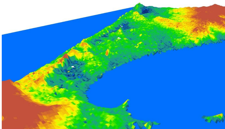
Figure 3 : vue en 3D du profil topographique des différents bassins versants dans les départements de Pikine et Guédiawaye (Modèle Numérique de Terrain, Extrait d'un exposé sur la «Contribution à l'identification des causes et à la recherche de solutions pour lutter contre les inondations » 1 , DGPRE 2009)
