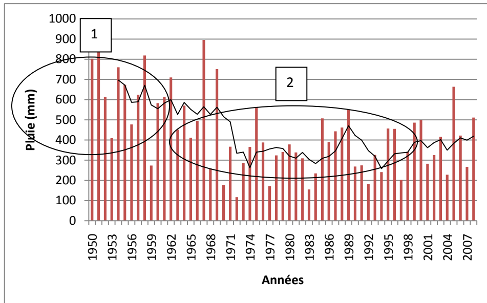
Figure 27 : pluviométrie annuelle à Dakar Yoff 1950-2008 (avec moyennes mobiles sur 5 ans) ; la période 1 correspond à une phase climatique humide, la période 2 à une phase sèche
